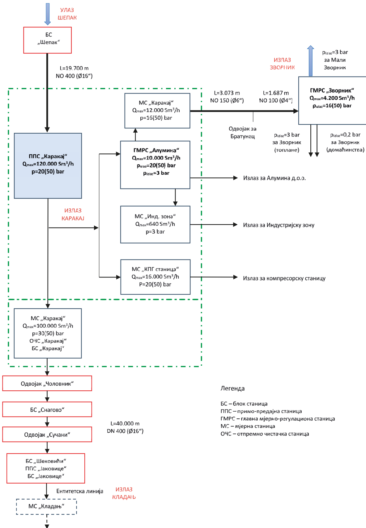
Шема транспортног система природног гаса Републике Српске
