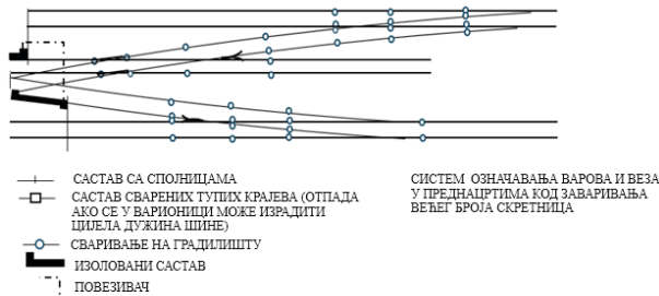
Слика 5. Скица плана заваривања више скретница
