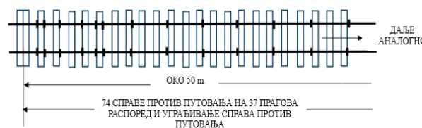
Слика 3. Скица постављања справа против уздужног путовања шина
