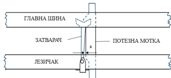
Слика 7. Дозвољено растојање затварача од потезне мотке на скретници
