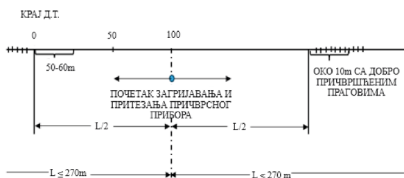
Слика 2. Графички нацрт продужења
