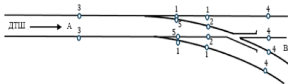
Слика 6. Редослед заваривања састава код скретница укључених у ДТШ
