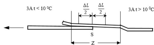
Слика 4. Скица прорачуна продужења мосних конструкција
